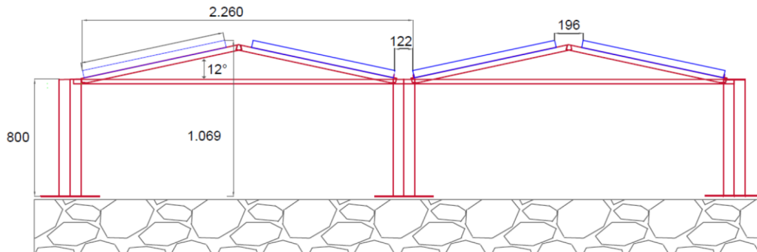
Abb. 3: Schematische Darstellung von den vorgesehenen PV-Modulen in Ost-Westausrichtung.
